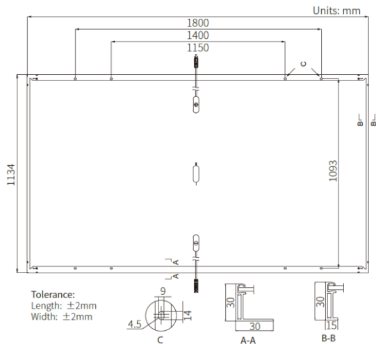
SBC MODULE STANDARD MODULE
